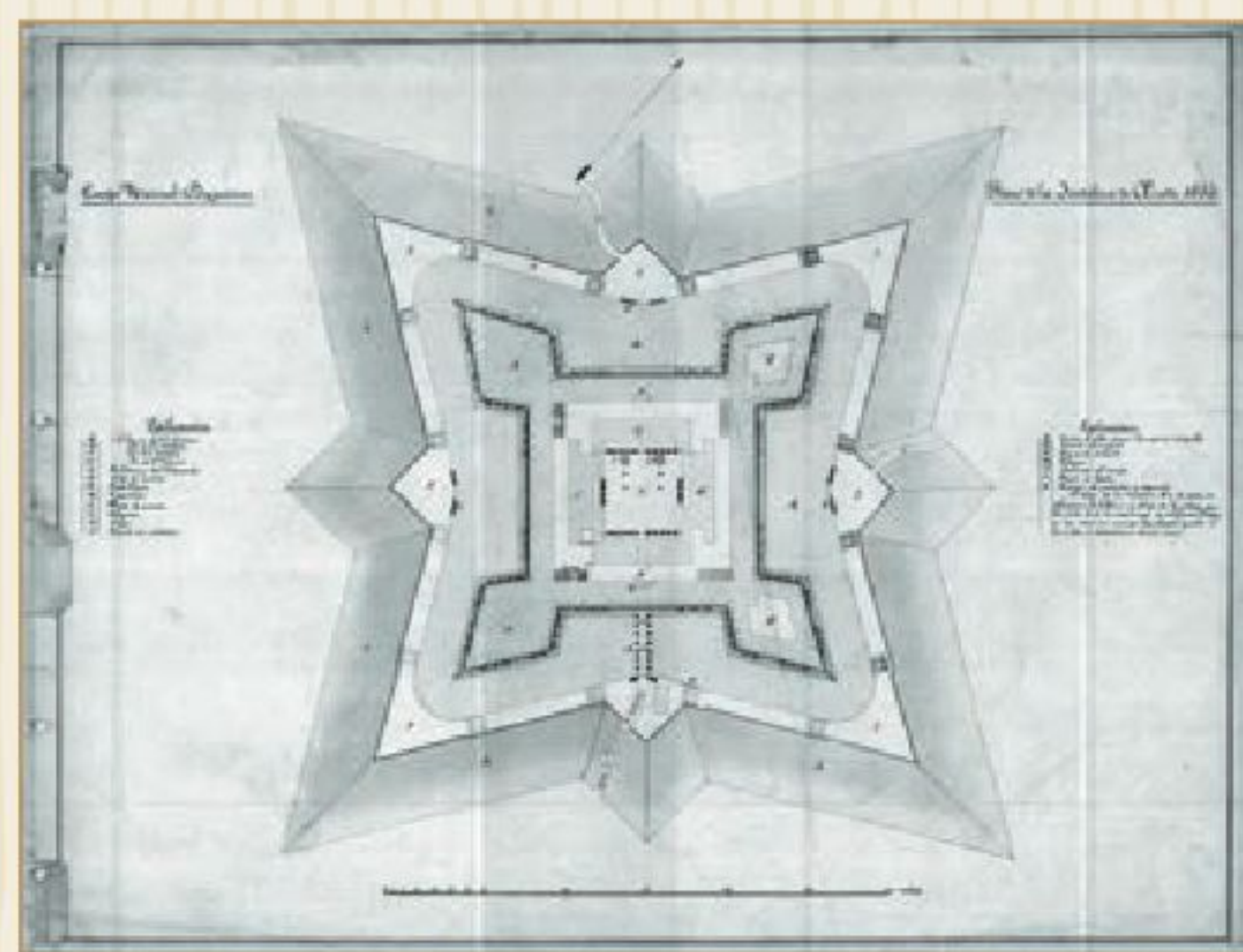
Plano de la fortaleza de San Carlos.
