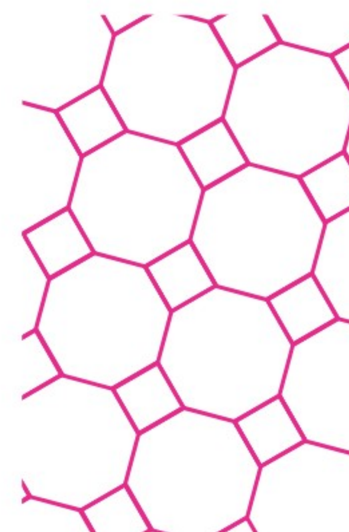
(4, 8^2)
