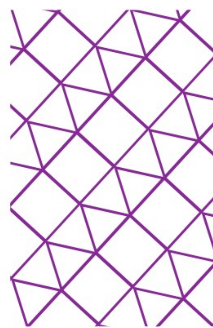
(3^3, 4^2)
