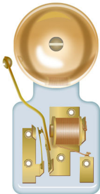
Figura 4.16 Componentes de un timbre eléctrico.
