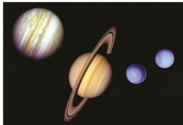
Figura 3.36 Planetas gaseosos del Sistema Solar.
