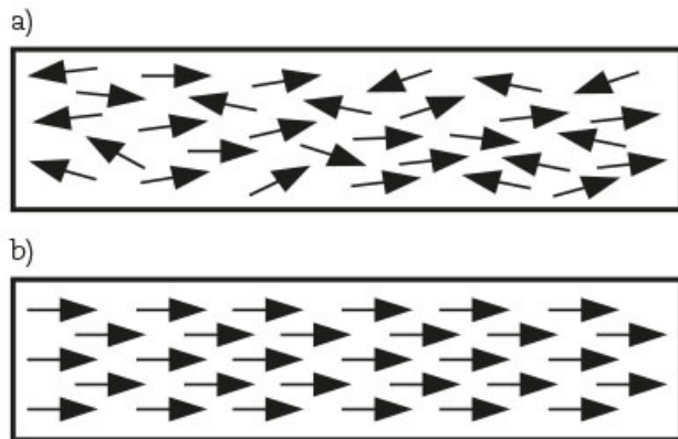
Figura 2.19 Observa el contraste entre la posición de los átomos de un objeto que no está en interacción con un imán (a) y el que sí tiene dicha interacción (b).
