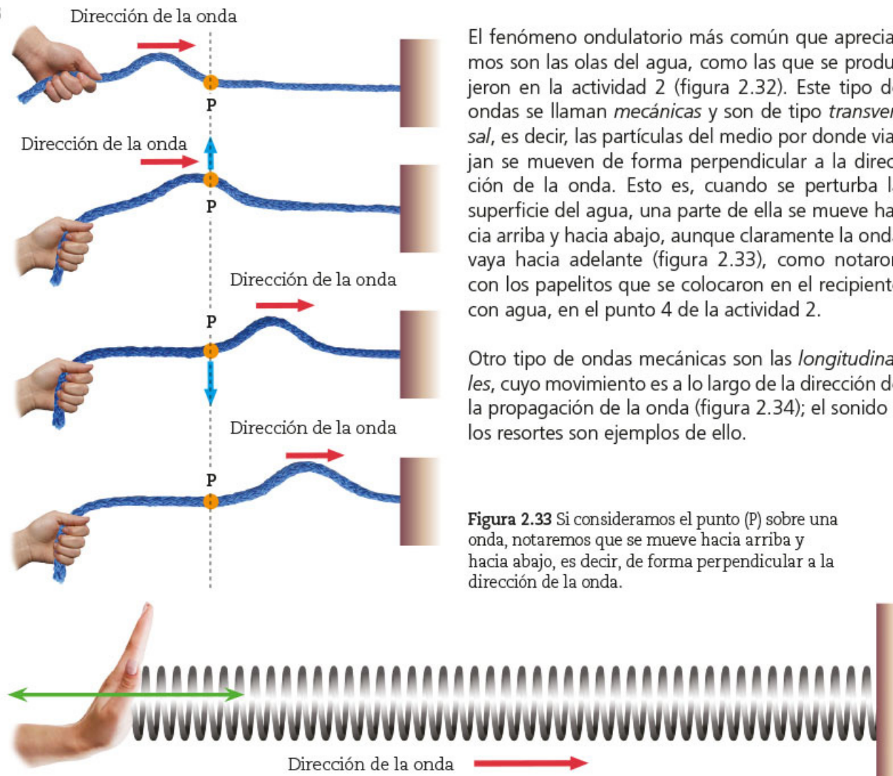
Figura 2.34 Al estirar o comprimir un resorte, se generan ondas longitudinales.
