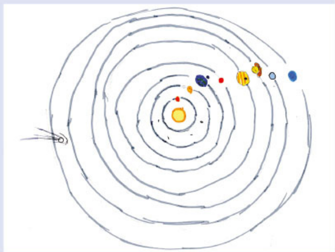
Dibujo del Sistema Solar elaborado por un estudiante.
