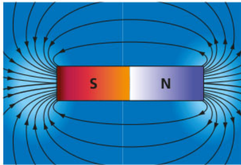
Figura 2.21 Se utilizan líneas o flechas para indicar el área de interacción del campo magnético. Las zonas donde el campo magnético tiene más fuerza se indican con líneas muy cercanas.
