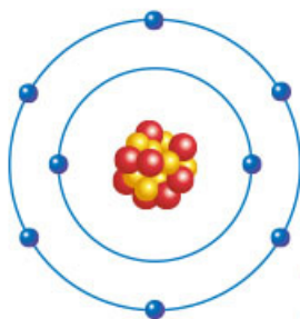
Figura 1.70 Si comparas ambos átomos, podrás identificar las diferencias entre el oxígeno y el cobre. Mencionalas.
