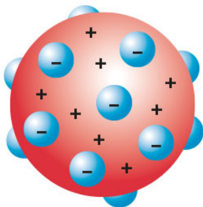
Figura 1.64 Representación gráfica del Modelo Atómico de Thomson.
