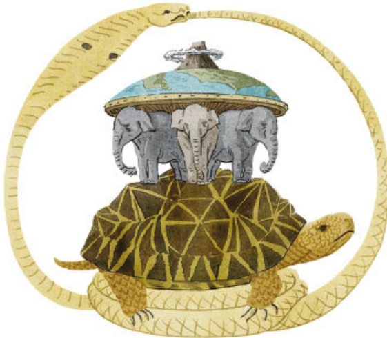
Figura 3.2 En algunas culturas de India se pensaba que ocurren temblores cuando los elefantes y la tortuga se mueven.
